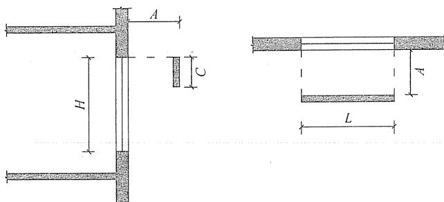
图 A-2 挡板遮阳参数 A 、 C 、 H 、 L 示意
