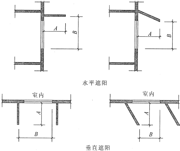
图 A-1 水平遮阳板和垂直遮阳板外挑参数 A、B 示意 A - 遮阳板外挑长度；B - 遮阳板根部到窗对边距离
