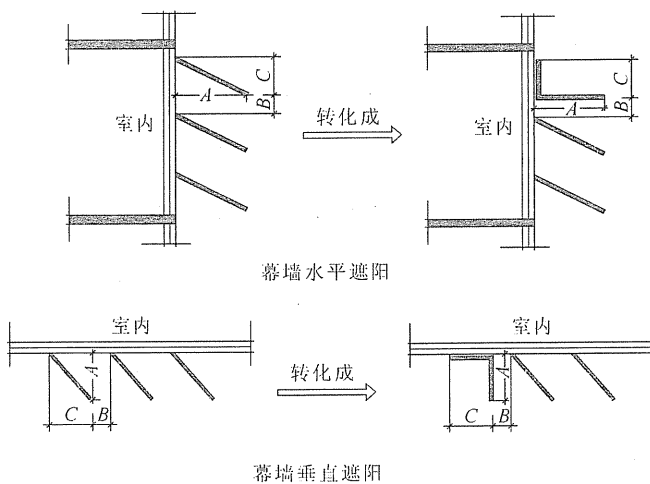
图 A-3 幕墙遮阳计算示意
