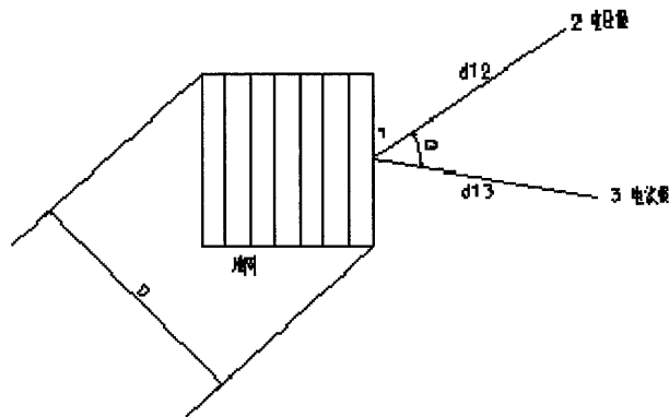
图 A.4 三角形布极图
