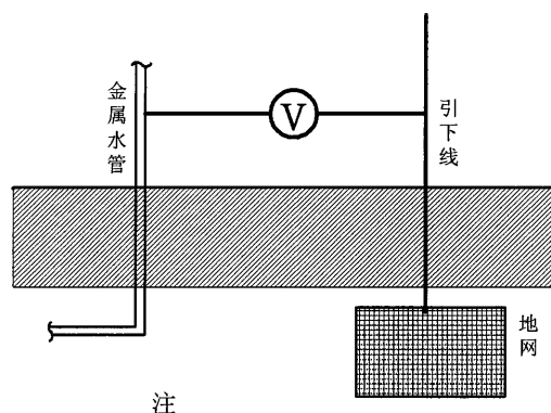
注 图 A.1 两点法测试原理示意图
