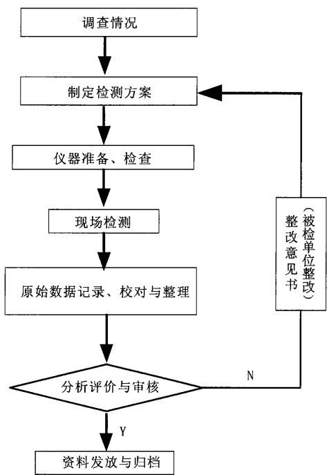
图 1 防雷装置检测流程图
