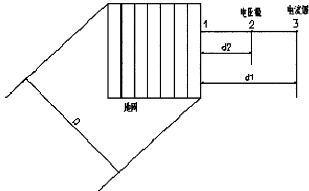
图 A.3 测量电极布置图
