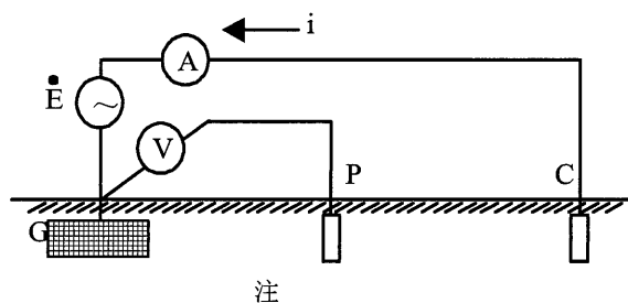
注 图 A.2 三极法测试原理图
