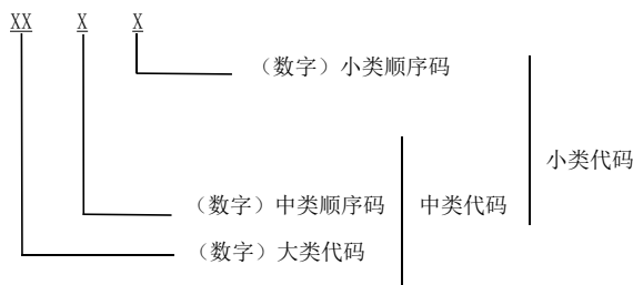
图2 代码结构图
