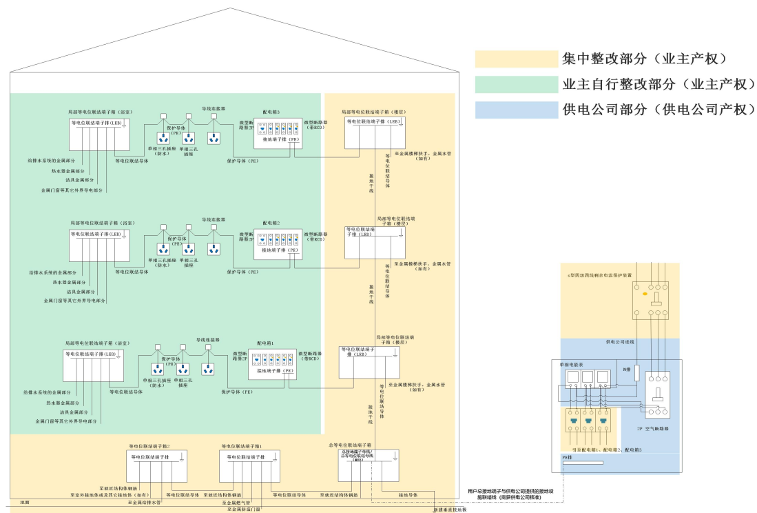
图 B.1 整改技术方案示意图 (A 方式)
