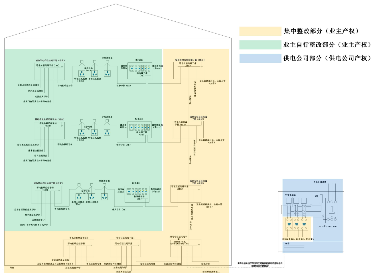
图 B.2 整改技术方案示意图 (B 方式)
