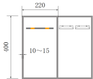
图 D.10 微型车位线（单位：cm）
