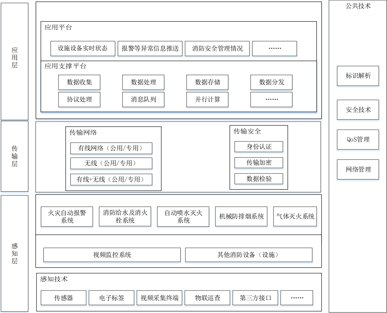
图1 系统架构图
