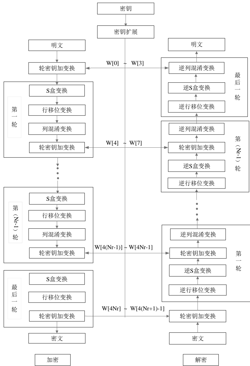
图 12 AES 加/解密过程图
