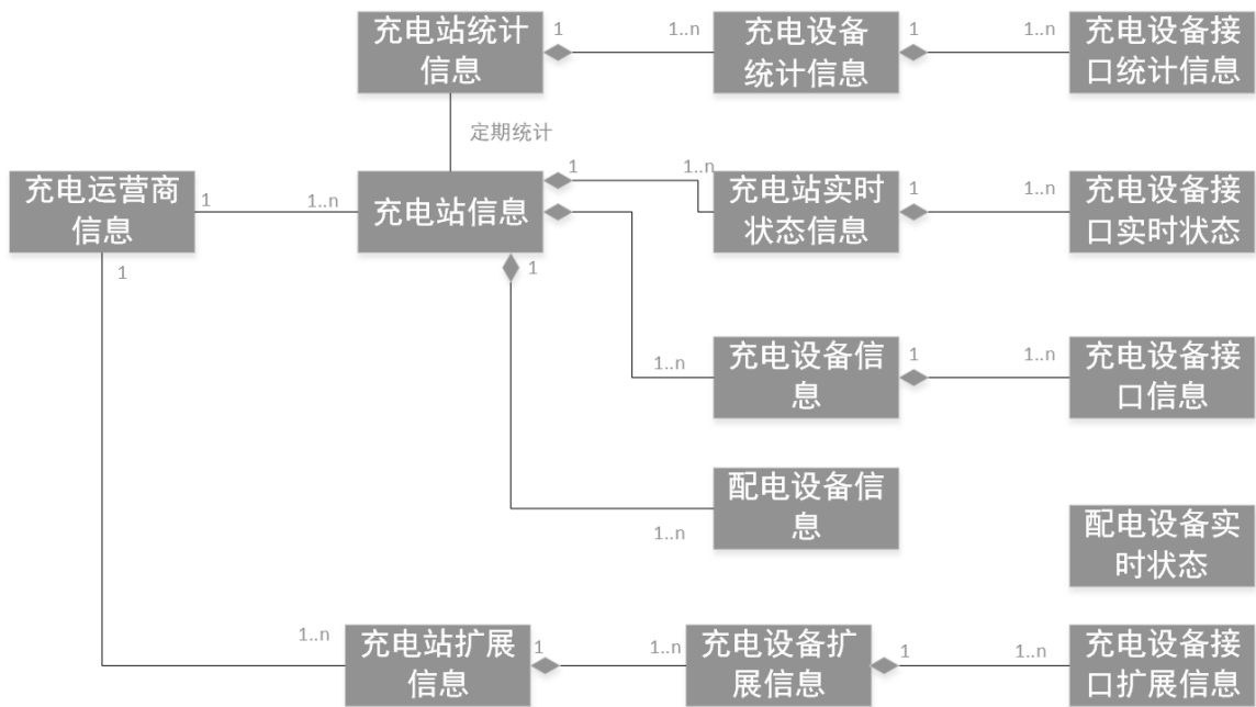
图 2 公共信息对象关系图
