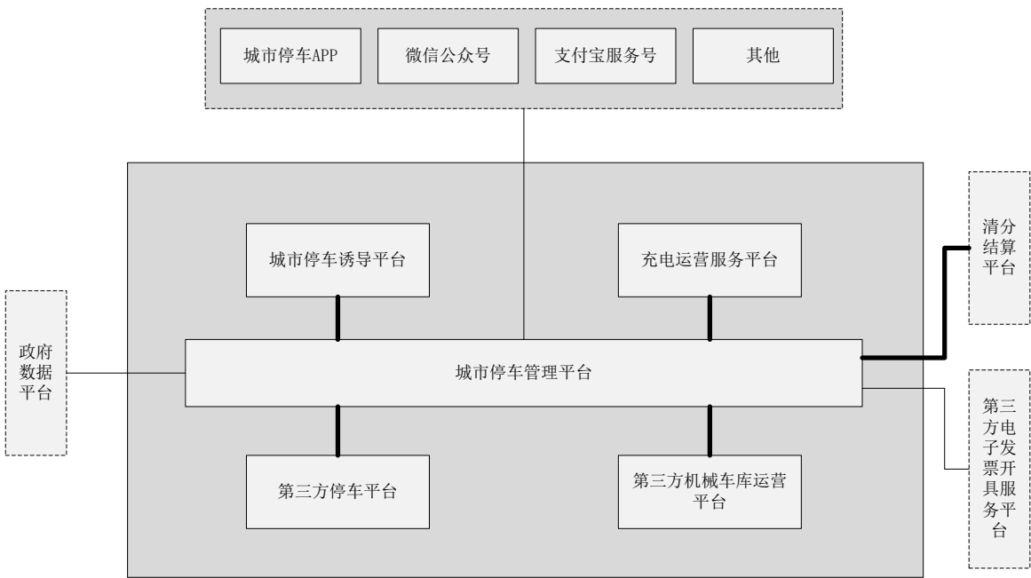
图1 城市停车管理平台架构图
