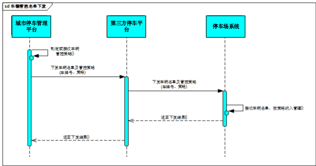
图 C.2 车辆管控名单下发业务流程图
