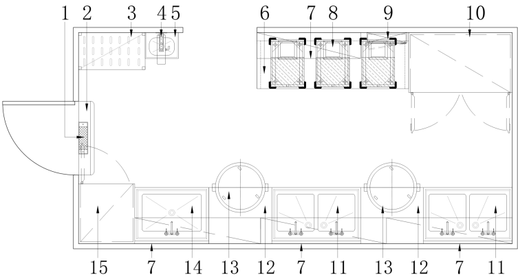
标序号说明： 1——灭蚊灯； 5——挂墙洗手星； 9——挂墙刀具消毒箱； 13——活动垃圾桶； 2——风幕机； 6——组合工作台； 10——四门高身雪柜； 14——大单星盆台； 3——可调节四层层架； 7——双层挂墙板； 11——双星盆台； 15——双门高身雪柜。 4——洗地龙头； 8——生料储存车； 12——单层工作台；
