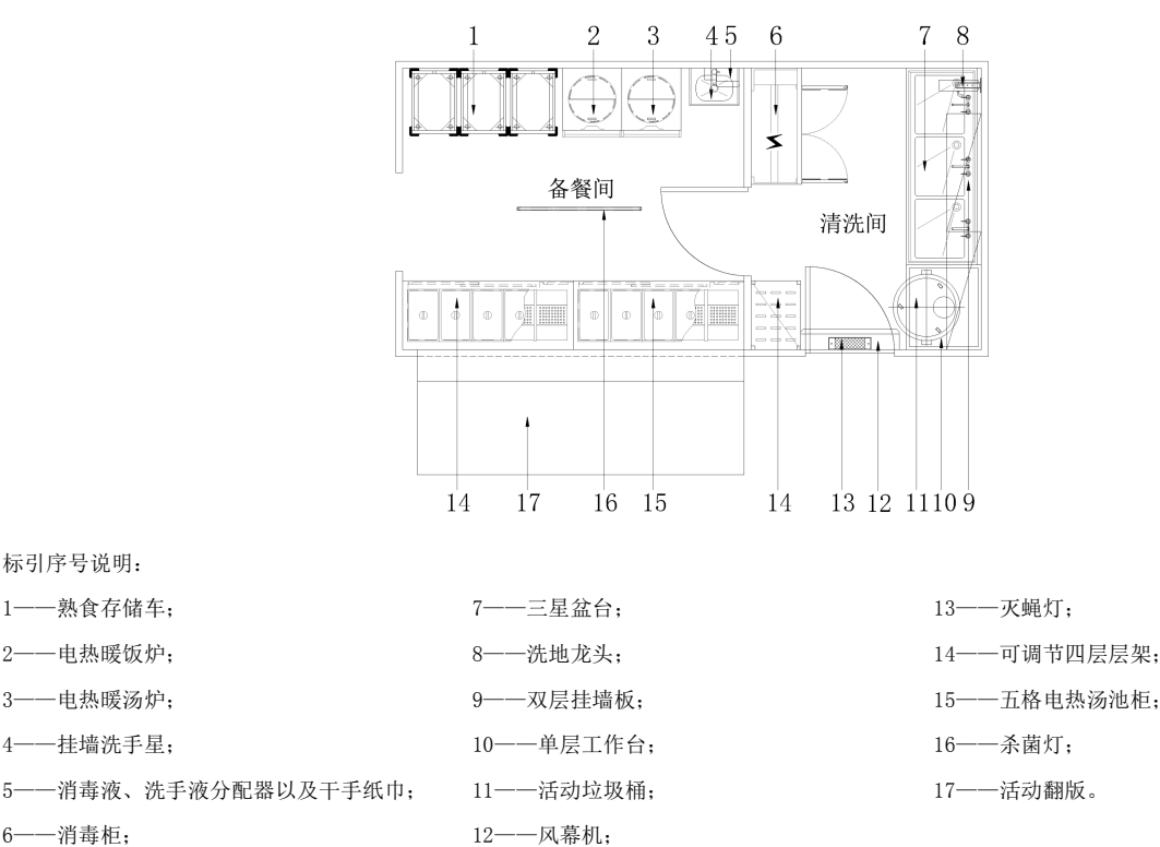
图 9 备餐/清洗厢体内部布局示意图
