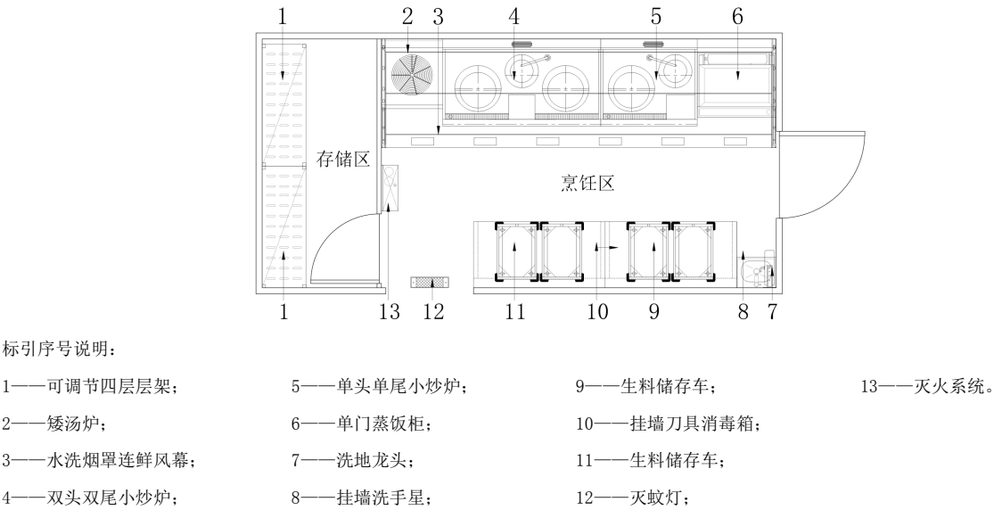
图 8 烹饪/存储厢体内部布局示意图
