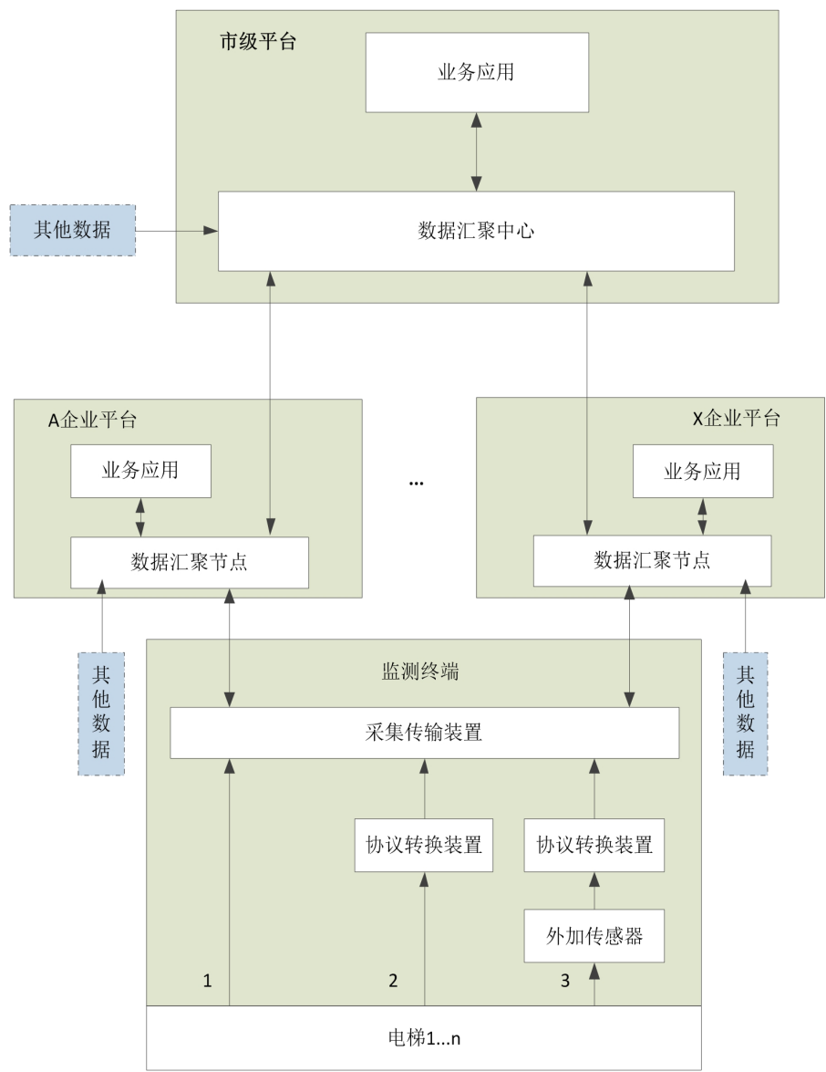
图 2 系统总体结构图
