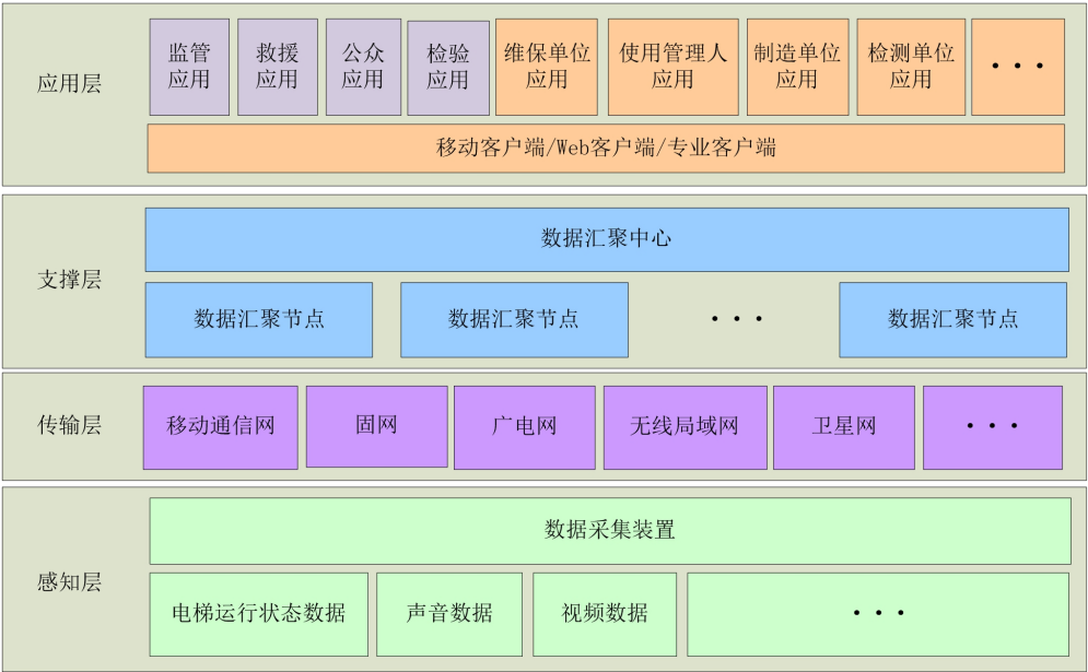
图 1 技术体系架构图
